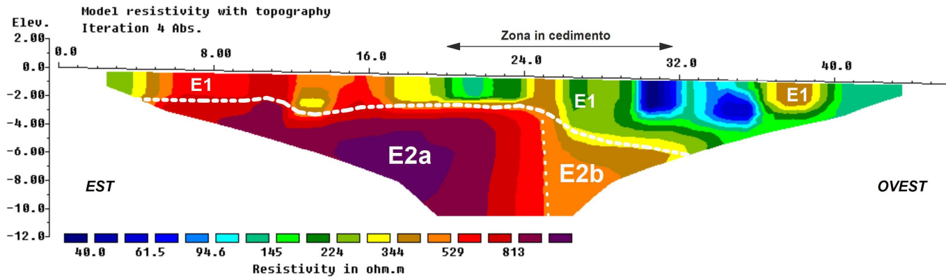
Sezione di resistività reale
