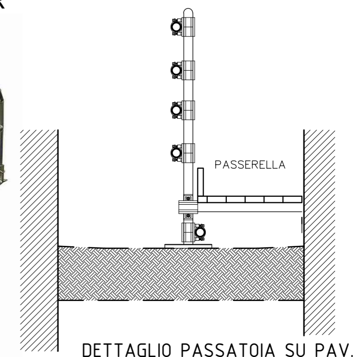
DETTAGLIO PASSATOIA SU PAV.
